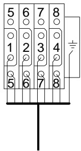
Câble de l'installation
