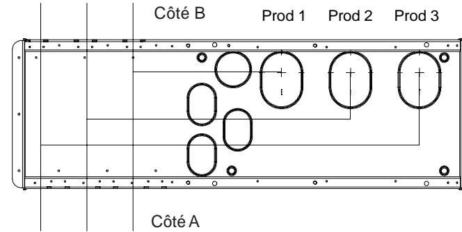
MODELES 3-3, 3-6, HS 3-3, HS 3-6
