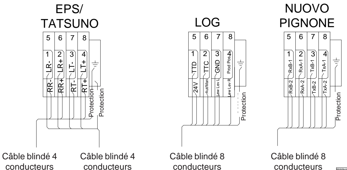
Câble de l'installation
